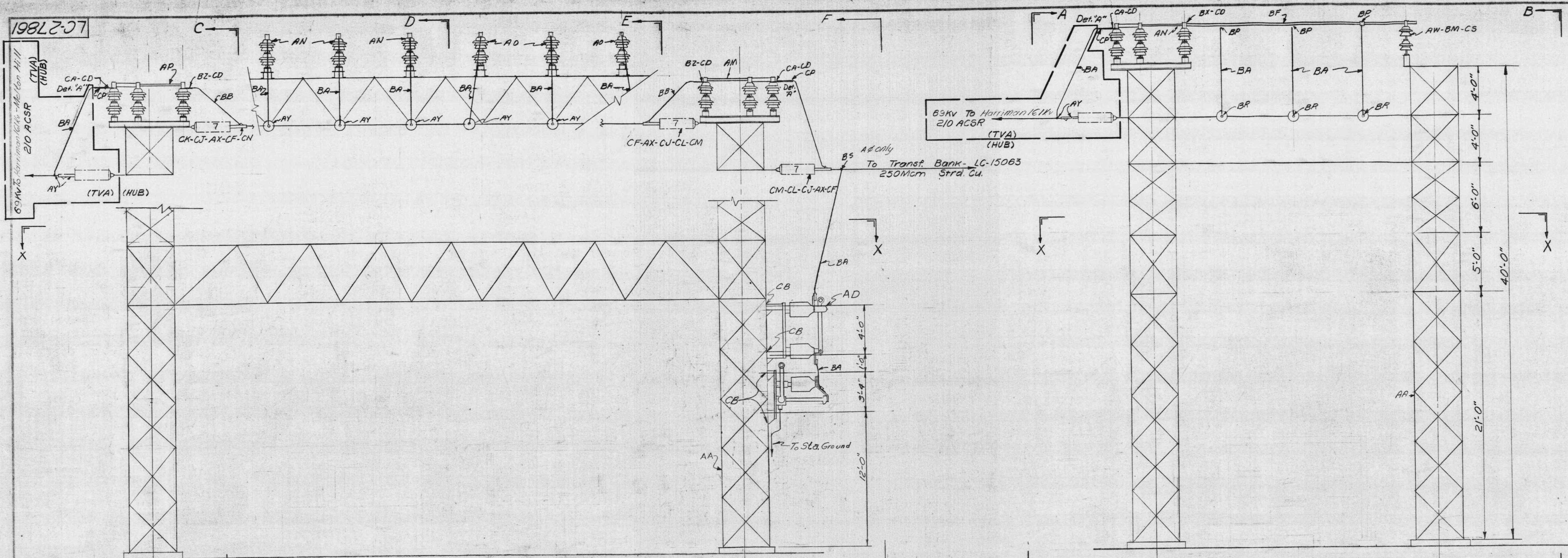
SECTION A-A
